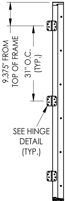
HINGE JAMB
